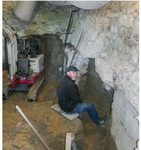
Guschaheimstall Curdin bei Unterfangungsarbeiten
